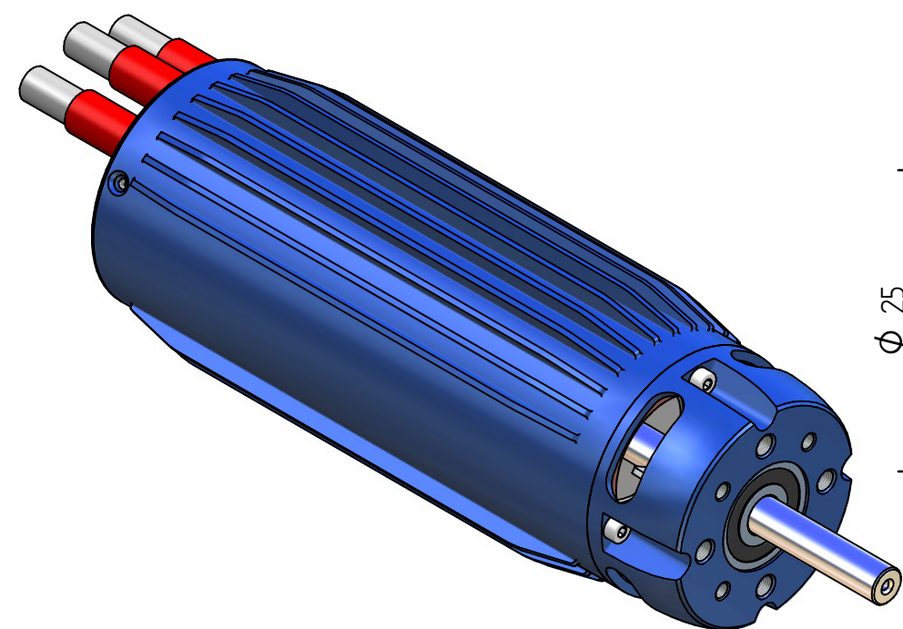
1:1 e-motor L-4075
