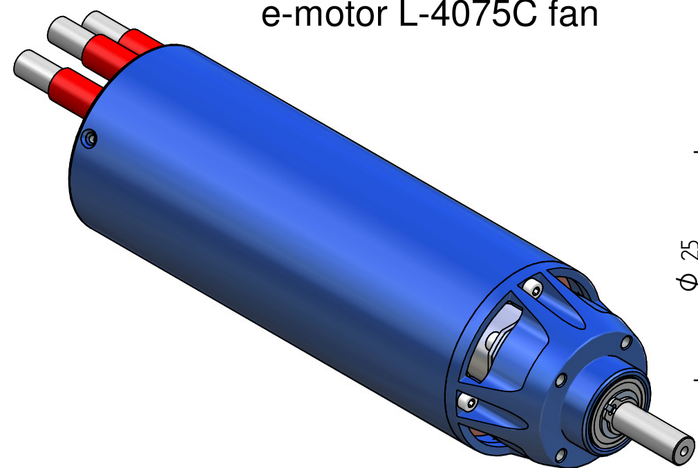
1:1 e-motor L-4075 gear
