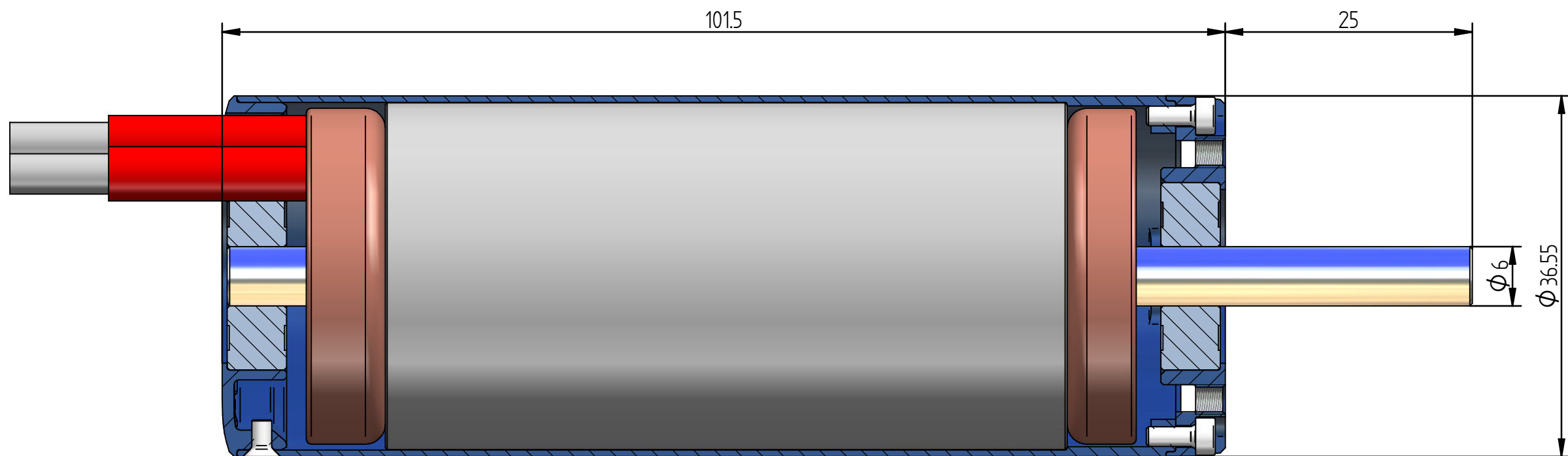
Schnitt A-A
