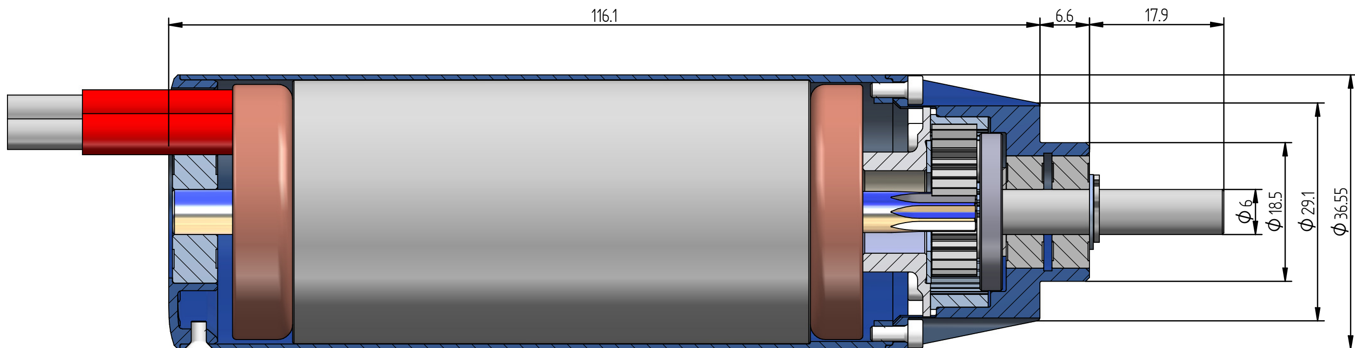
Schnitt B-B
