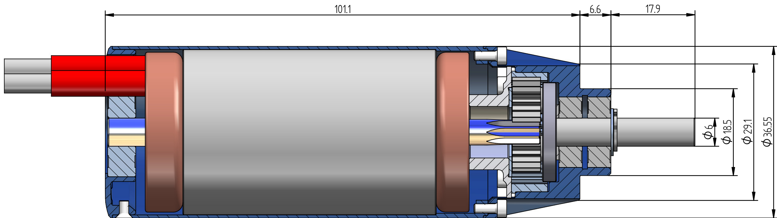
Schnitt B-B
