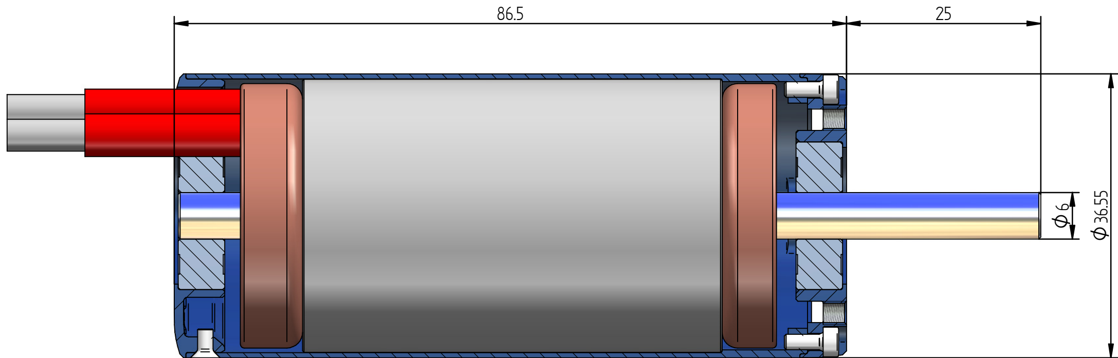
Schnitt A-A
