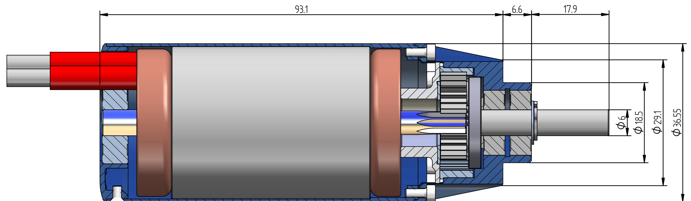
Schnitt B-B
