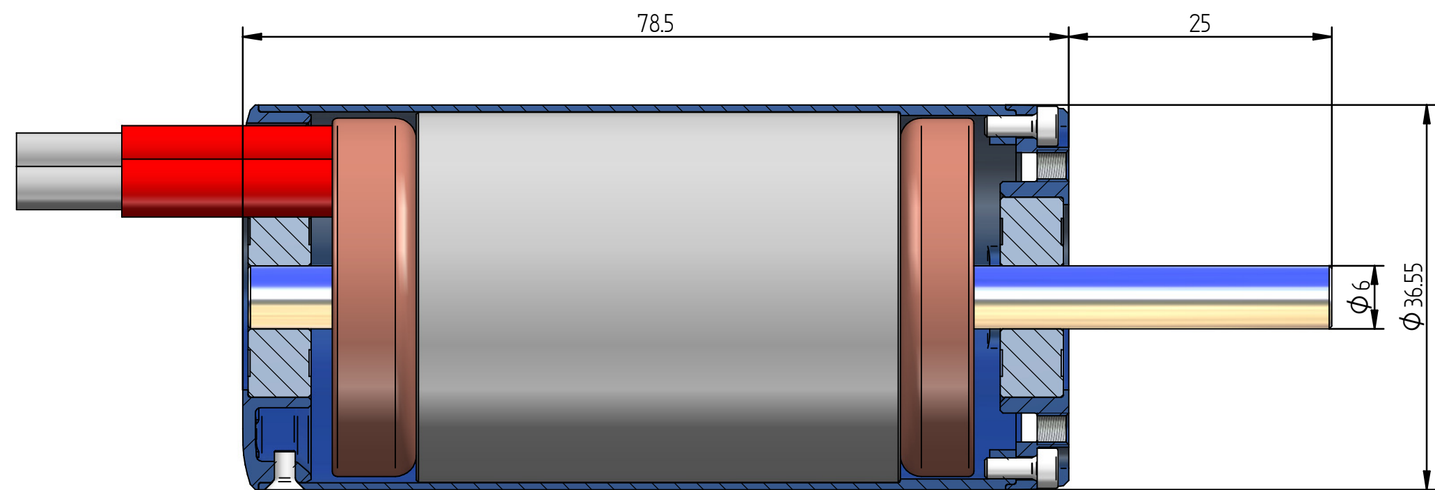
Schnitt A-A
