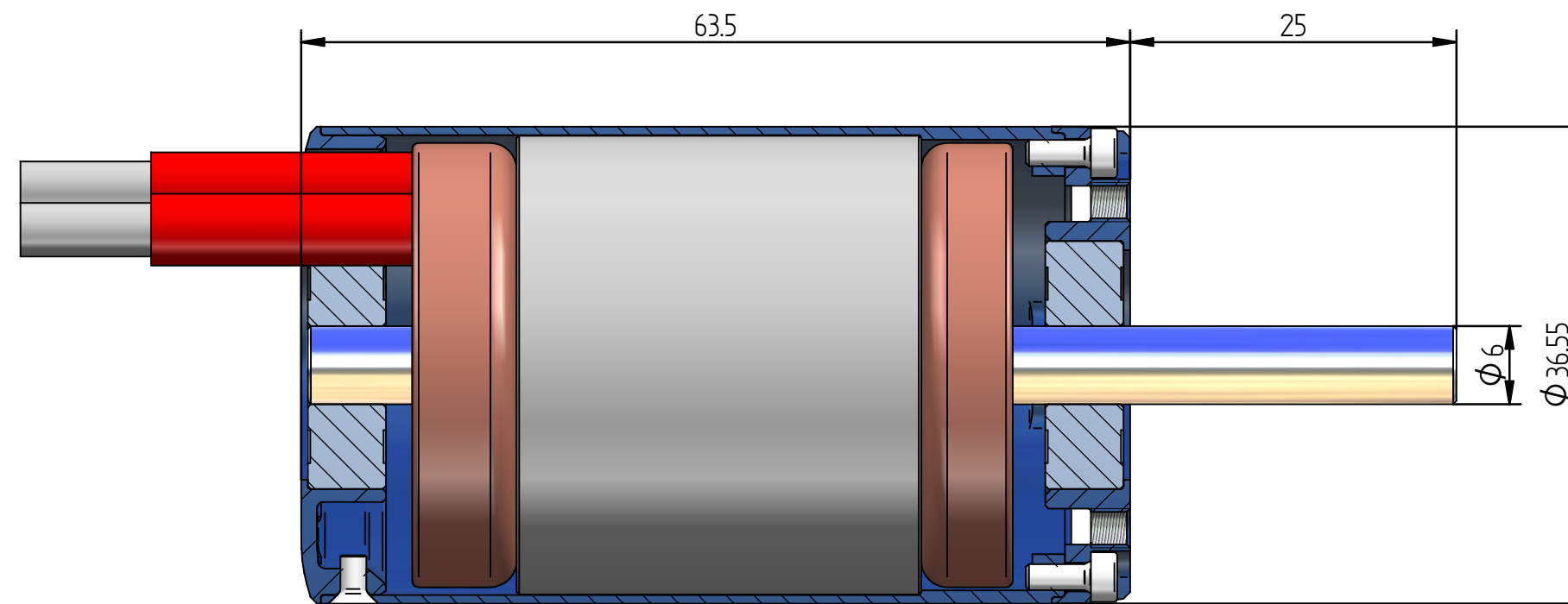
Schnitt A-A
