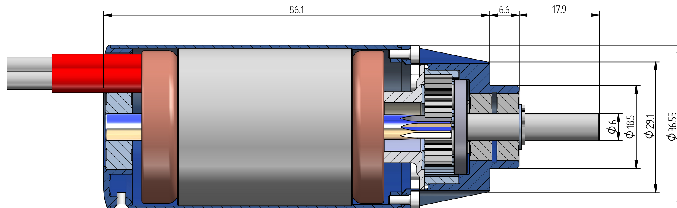
Schnitt B-B
