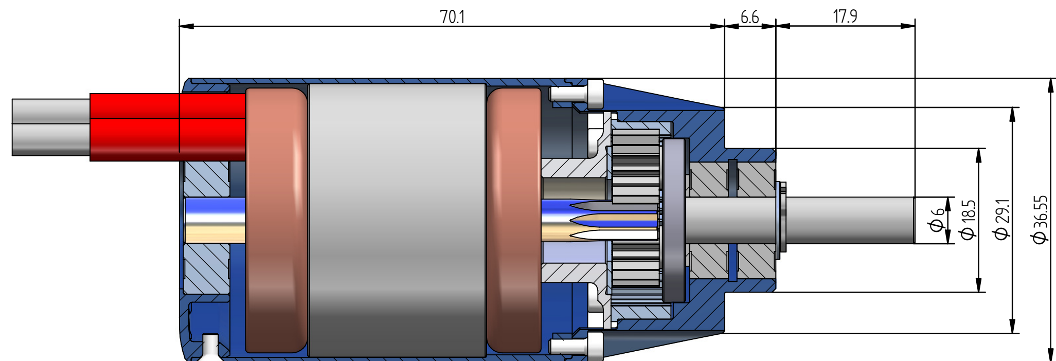
Schnitt B-B
