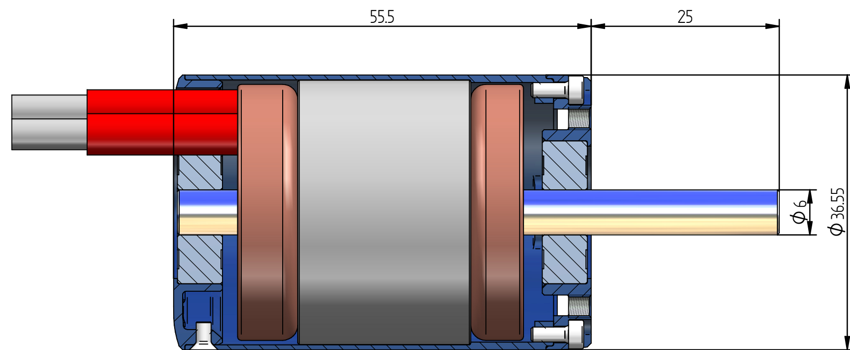
Schnitt A-A
