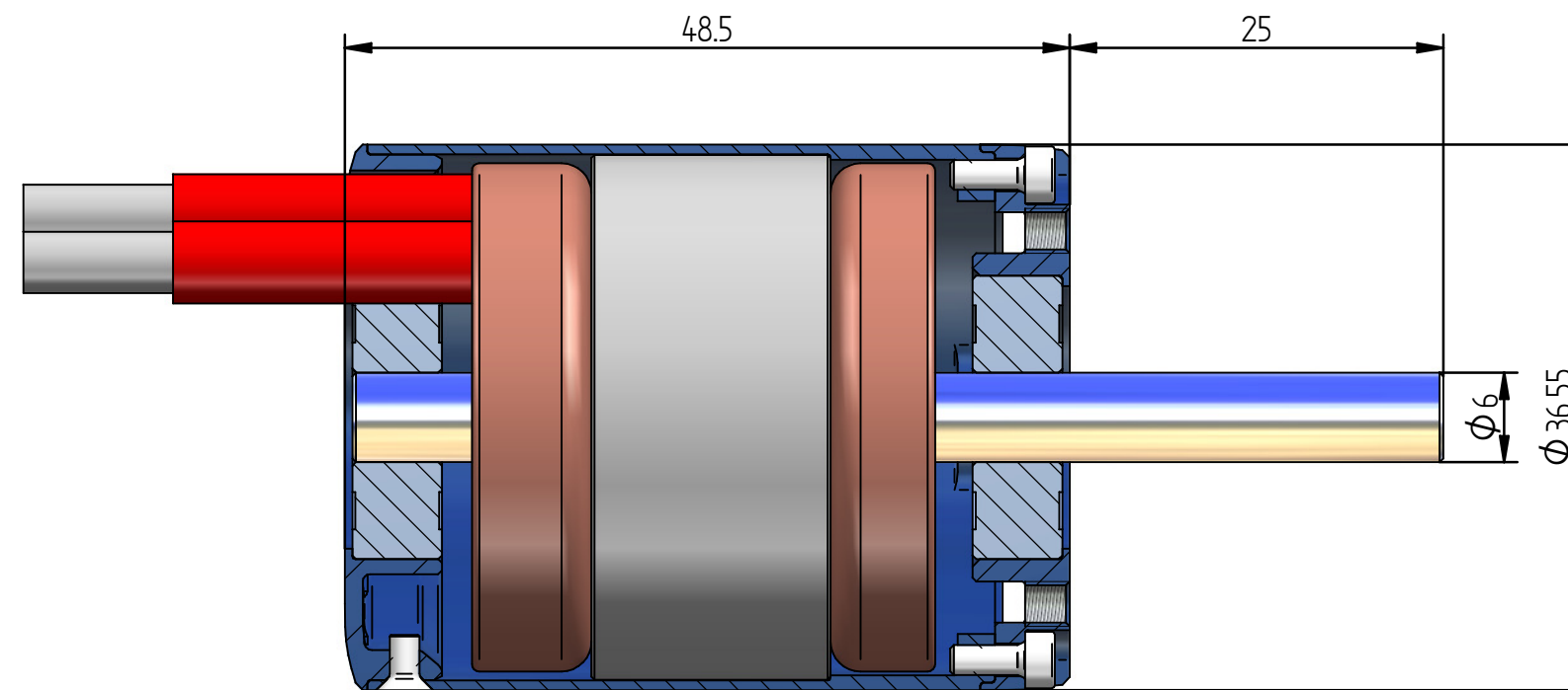
Schnitt A-A
