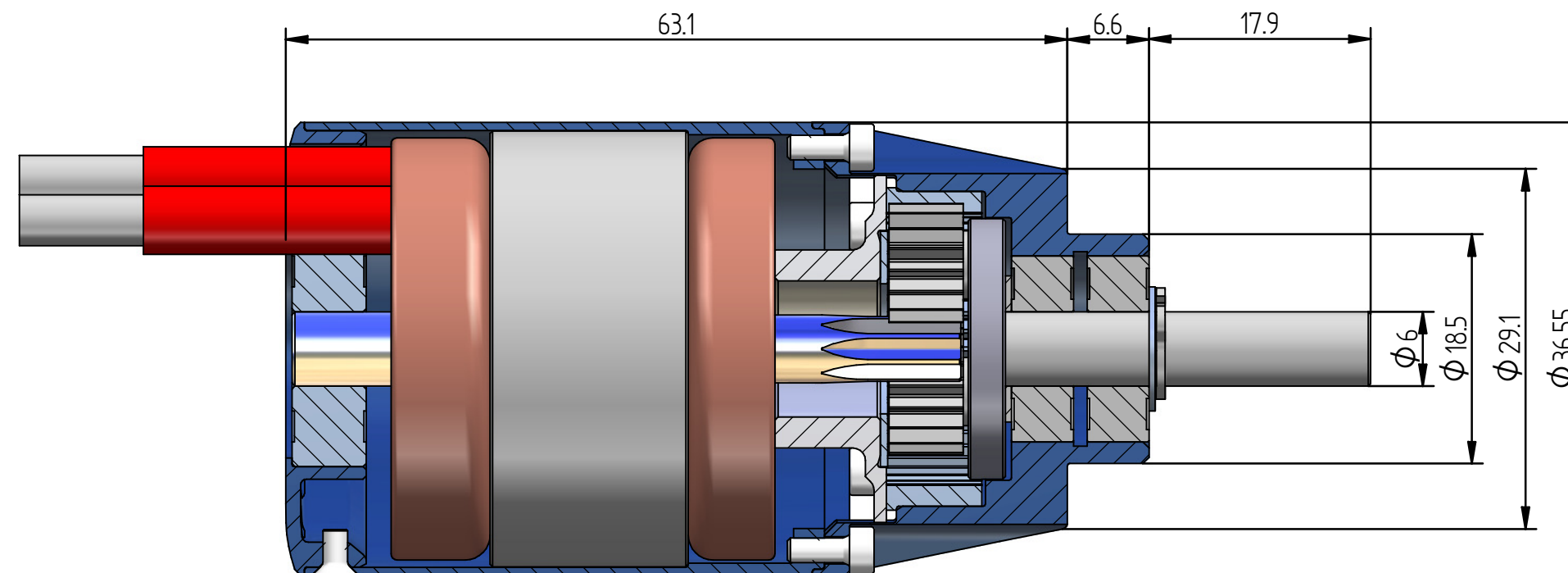
Schnitt B-B
